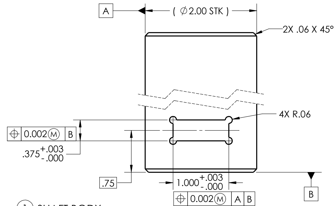
① SHAFT BODY SCALE 1:1
