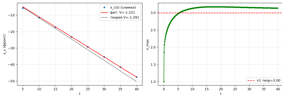
Рисунок 3.2 — Траектория фронта x_c(t) (линейный участок даёт скорость фронта V ) и эволюция концентрации n_{\max}(t) .
