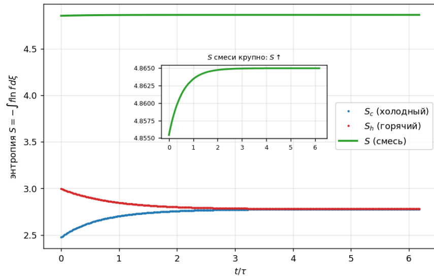
Рисунок 2.8 — Энтропии: суммарная энтропия смеси монотонно возрастает ( H -теорема); компоненты ведут себя противоположно.
