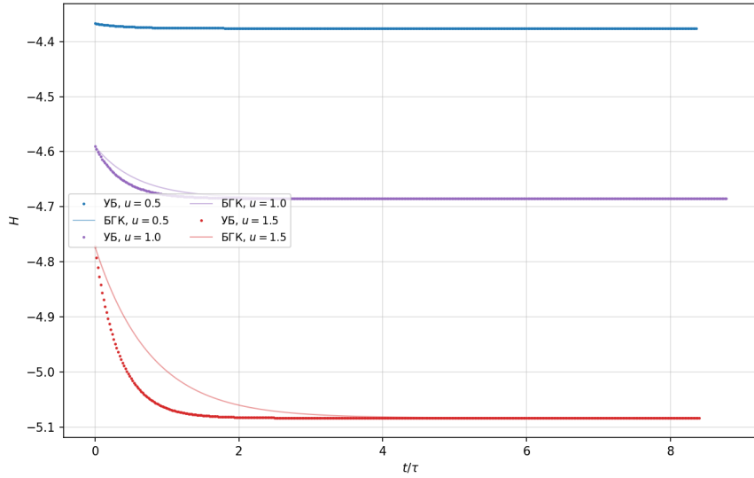
Рисунок 2.3 — Эволюция H -функции Больцмана: монотонное невозрастание ( H -теорема).
