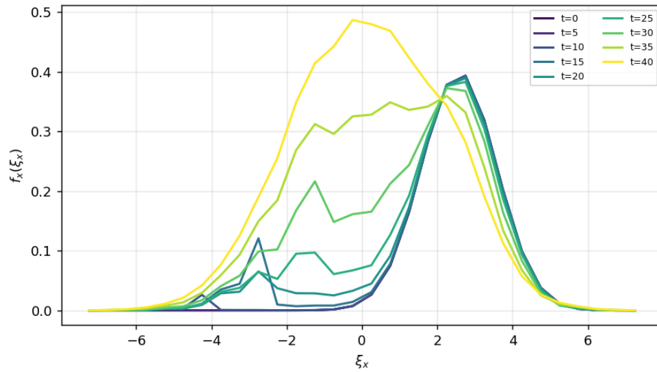
Рисунок 3.3 — Эволюция f_x(\xi_x) в середине области: переход от холодного набегающего потока (пик при \xi_x \approx u_0 ) к послескачковому распределению.
