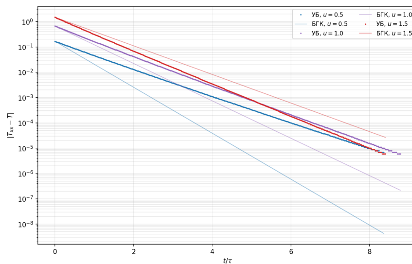
Рисунок 2.2 — Затухание анизотропии |T_{xx} - T| в логарифмическом масштабе в сравнении с моделью БГК.
