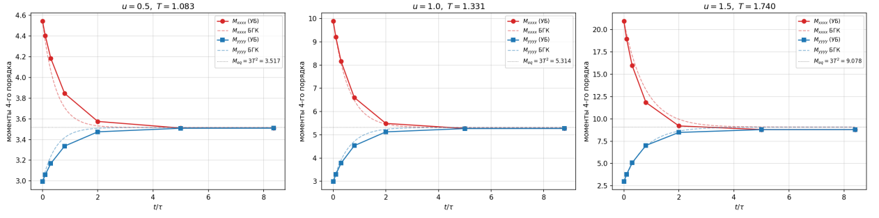
Рисунок 2.4 — Продольный M_{xxxx} и поперечный M_{yyyy} моменты 4-го порядка: многомодовость релаксации против модели БГК (пунктир).
