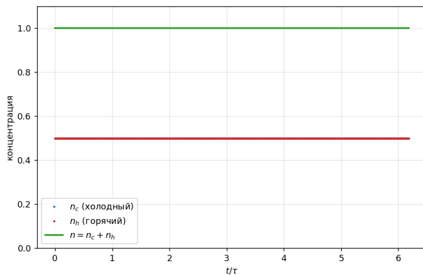
Рисунок 2.7 — Сохранение концентраций компонент n_c = n_h = 0,5 (контроль метода).
