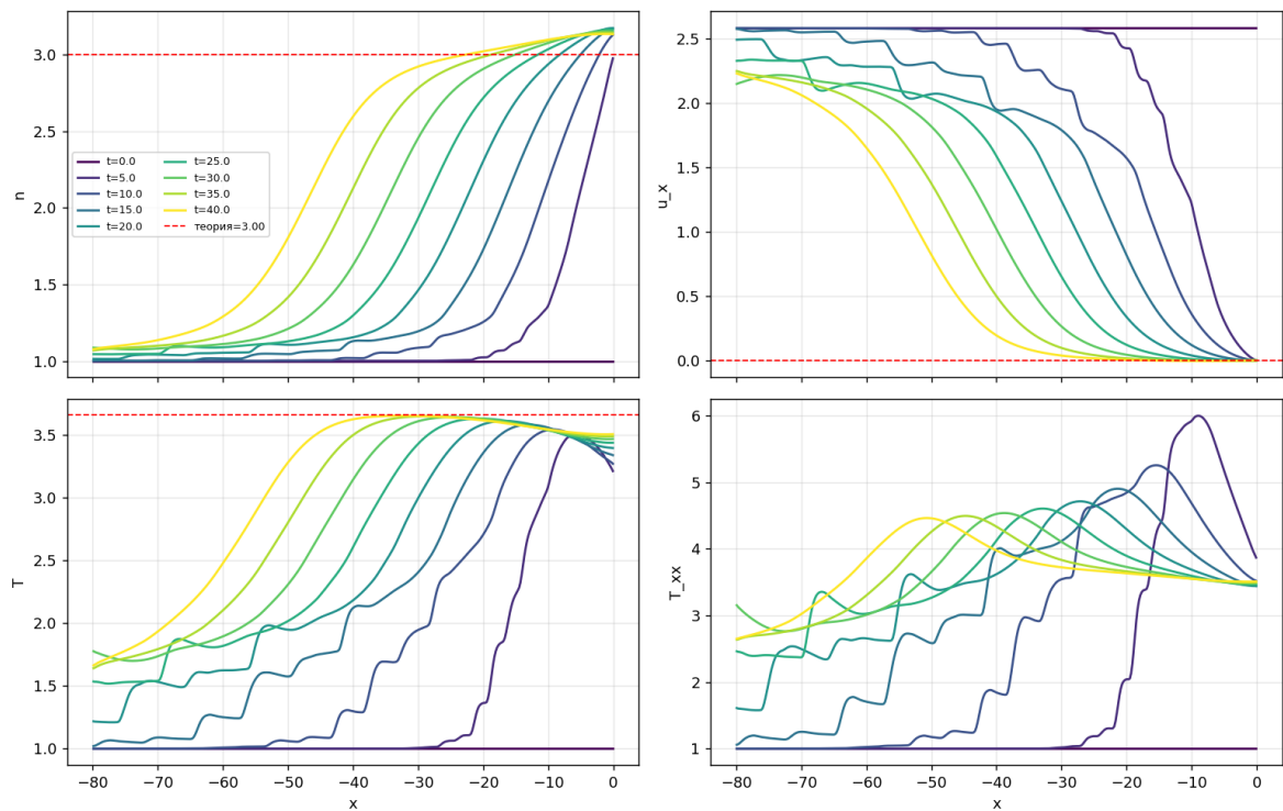
Рисунок 3.1 — Профили макропараметров n , u_x , T , T_{xx} вдоль оси x в различные моменты времени (установившаяся ударная волна).
