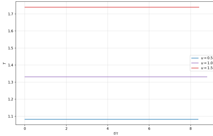
Рисунок 2.1 — Эволюция температуры T(t) для трёх значений u : общая температура сохраняется (контроль энергии).
