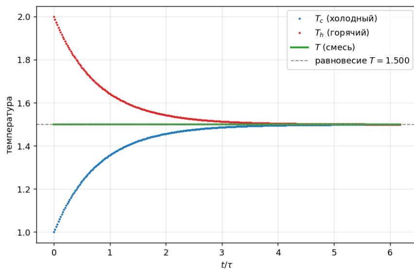
Рисунок 2.6 — Выравнивание парциальных температур T_c и T_h к общему значению T_{eq} = 1,5 .
