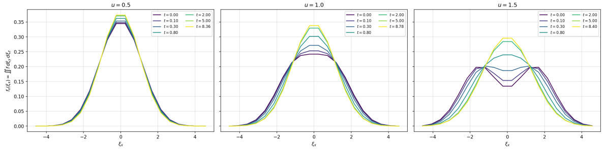
Рисунок 2.5 — Эволюция одномерной функции распределения f_x(\xi_x) от двугорбой к равновесной максвелловской.
