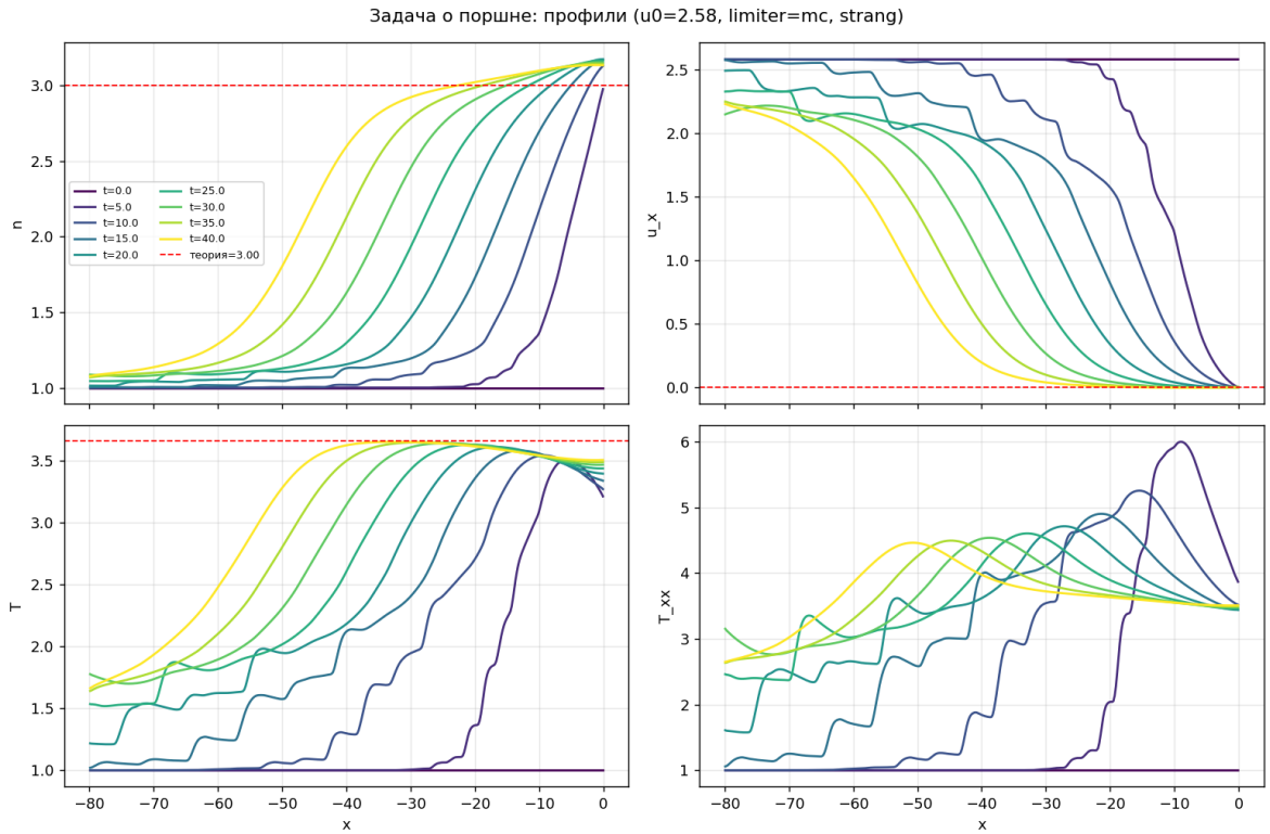
Рисунок 3.1 — Профили макропараметров n , u_x , T , T_{xx} вдоль оси x в различные моменты времени (установившаяся ударная волна, конфигурация L = 80 , N_x = 400 ).
