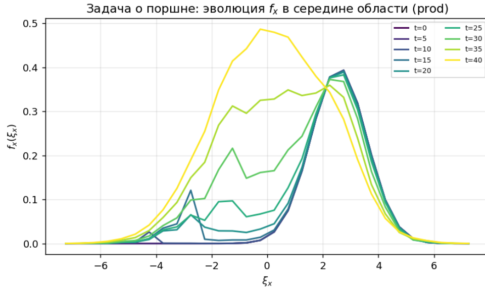
Рисунок 3.3 — Эволюция f_x(\xi_x) в середине области: переход от холодного набегающего потока (пик при \xi_x \approx u_0 ) к послескачковому распределению ( \xi_x \approx 0 ).
