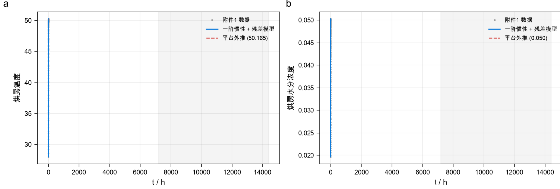
图 3 烘房环境的一阶惯性辨识。数据点、辨识模型与平台期统计区间（阴影）。左：温度 ( R^2 = 0.9973 , \tau = 1776 \text{ s} )；右：水分浓度 ( R^2 = 0.9944 , \tau = 2522 \text{ s} )。
