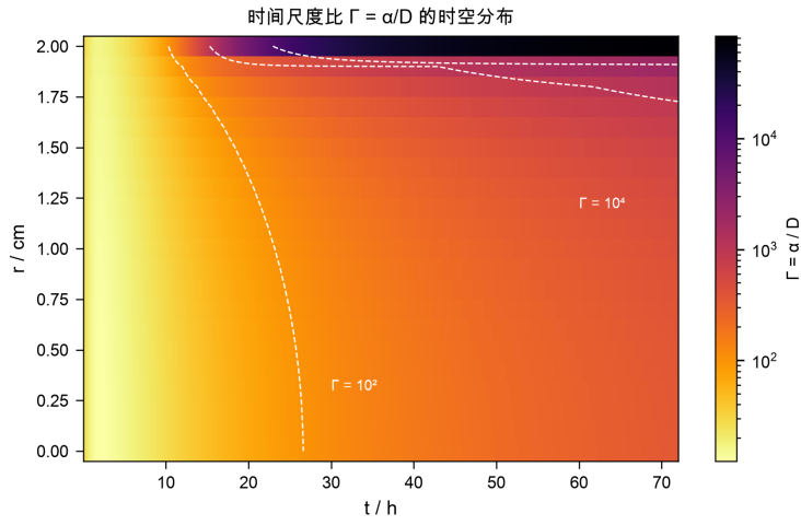
图 8 时间尺度比 \Gamma = \alpha/D 的时空分布（对数色标，虚线为等值线）。湿态 \Gamma \sim 10 、干态 \Gamma \sim 10^5 ：热湿耦合强度随干燥进程衰减。
