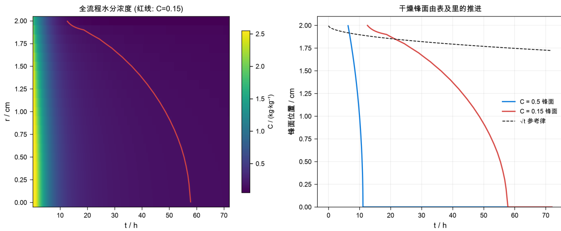
图 10 全流程水分浓度（左：二维热图，横轴为时间；右： C=0.5 与 C=0.15 的干燥锋面位置随时间的变化，虚线为 \sqrt{t} 参考）。锋面由表及里推进，早期近似扩散平方根律，晚期受 D 下降影响减速。
