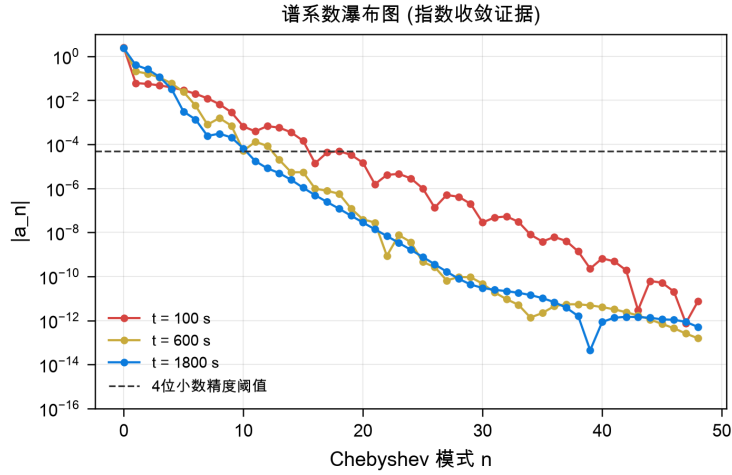
图 5 谱系数随模式数指数衰减 ( t = 1800 \text{ s} )。末位系数 5 \times 10^{-13} 远低于 4 位小数精度阈值 5 \times 10^{-5} 。
