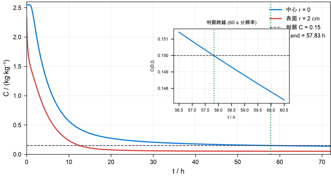
图 9 烘干时长判定。72 h 中心/表面含水率轨迹与 0.15 判据线，内嵌 56.5–60.5 h 放大图显示 60 s 分辨率下的跨越过程。
