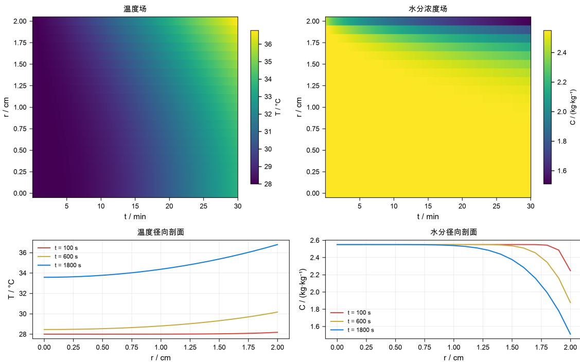
图 6 预热阶段时空演化 (二维热图, 上) 与典型时刻径向剖面 (下)。左列温度, 右列水分浓度。
