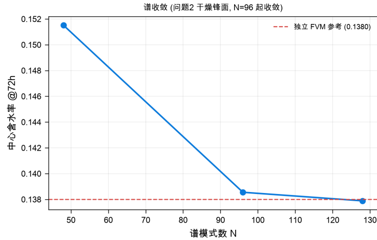
图 7 空间收敛：72 h 中心含水率随谱模式数的变化。 N = 48 欠分辨， N = 96 起与独立有限体积法参考解（虚线）一致。
