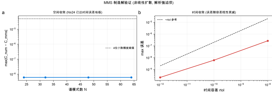
图 13 制造解验证。(a) 空间： N \geq 24 后谱误差低于时间误差水平；(b) 时间：误差随容差线性衰减。
