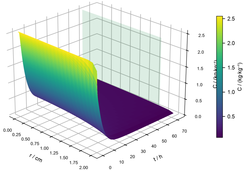
图 11 全流程水分浓度的三维曲面 (图 10 左图的立体视角): 红色曲线为 C = 0.15 等值线在曲面上的轨迹, 绿色半透明面为烘干结束时刻 t_{end} = 57.83 \text{ h} 的截面。
