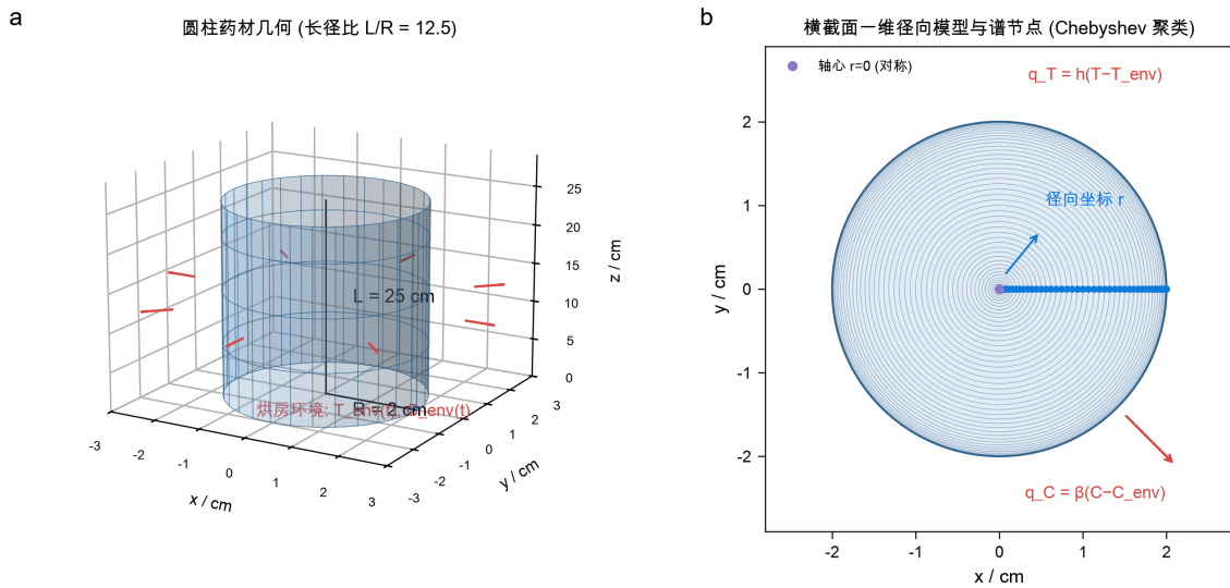
图 1 圆柱药材的几何模型与一维径向离散。(a) 圆柱几何（长 25 cm 、半径 2 cm ，长径比 12.5 ），烘房环境经对流传热传质作用于表面；(b) 横截面上的一维径向模型：径向坐标 r 、轴心对称条件与表面 Robin 边界，谱配点节点在表面与轴心处聚类。
