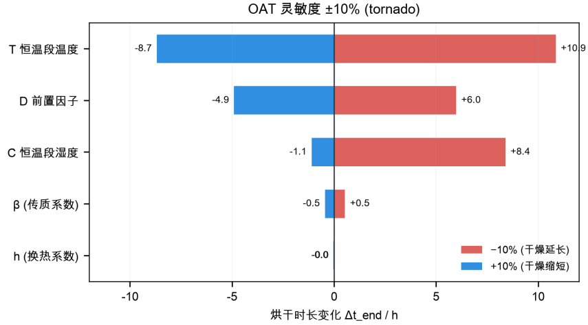
图 14 灵敏度 tornado 图。恒温段温度为主导控制量，换热系数影响可忽略。
