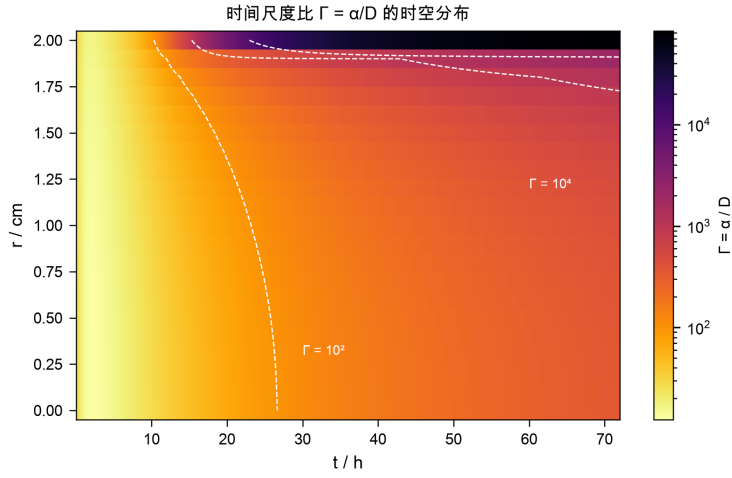
图 8 时间尺度比 \Gamma = \alpha/D 的时空分布（对数色标，虚线为等值线）。湿态 \Gamma \sim 10 、干态 \Gamma \sim 10^5 ：热湿耦合强度随干燥进程衰减。
