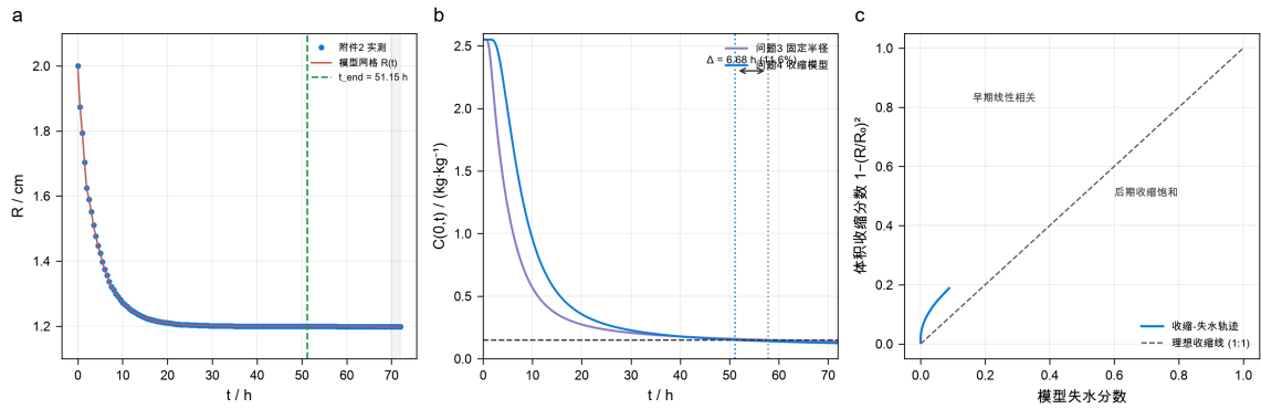
图 9 收缩干燥：(a) 附件 2 实测半径与模型网格轨迹；(b) 问题三与问题四中心含水率对比， \Delta t_{end} = 6.68 \text{ h} （11.6%）；(c) 收缩-失水一致性检验：早期线性相关（收缩由失水驱动），后期收缩趋于饱和（骨架结构抵抗压实），与附件 2 的 70 h 收缩平台一致。
