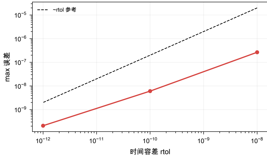
时间收敛 (误差随容差线性衰减)
