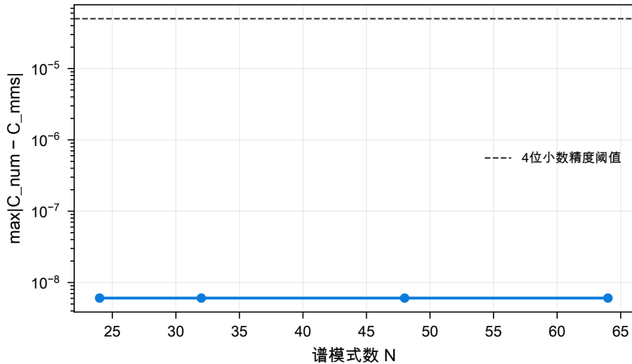
空间收敛 (N≥24 已达时间误差地板)
