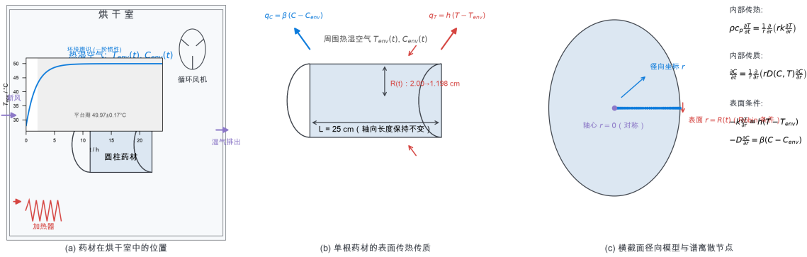
图 1 物理机理示意图。(a) 药材在烘干室中的位置与环境辨识（内嵌：环境温度的一阶惯性拟合与平台期）；(b) 单根药材的表面传热传质（轴向长度不变、半径收缩至 R(t) ）；(c) 横截面径向模型：控制方程、边界条件与谱配点节点（表面与轴心处聚类）。
