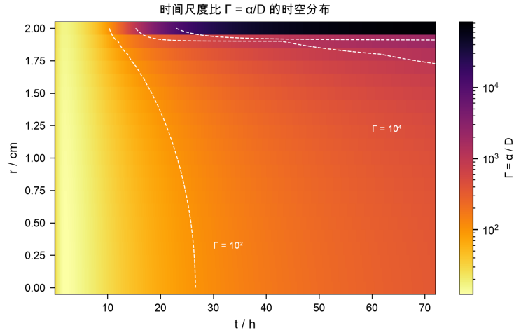
图 8 时间尺度比 \Gamma = \alpha/D 的时空分布（对数色标）。 \Gamma 增大表示热扩散相对水分扩散更快，温度场更快趋于准稳态。
