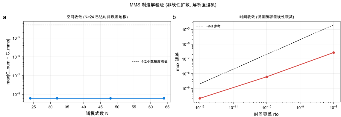
图 12 制造解验证。(a) 空间： N \geq 24 后谱误差低于时间误差水平；(b) 时间：误差随容差线性衰减。
