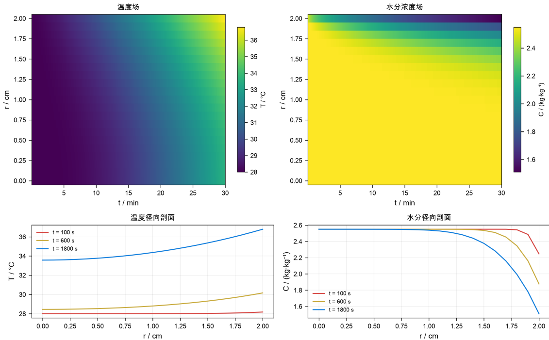
图 6 预热阶段时空演化 (二维热图, 上) 与典型时刻径向剖面 (下)。左列温度, 右列水分浓度。
