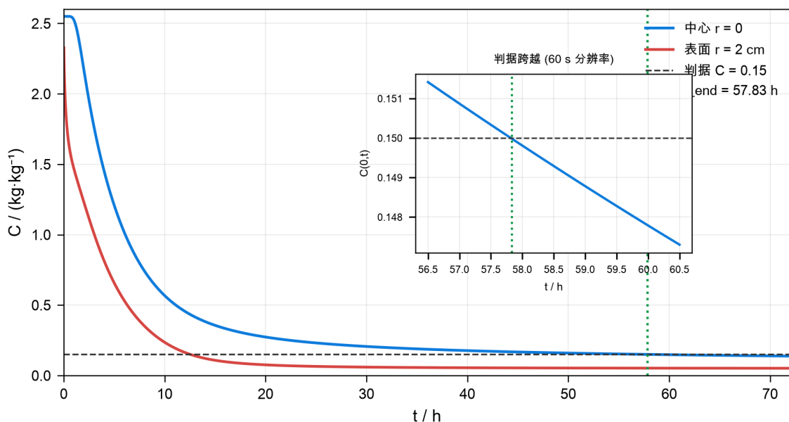
图 9 中心/表面含水率轨迹与 0.15 判据线 (内嵌 56.5–60.5 h 放大图)。
