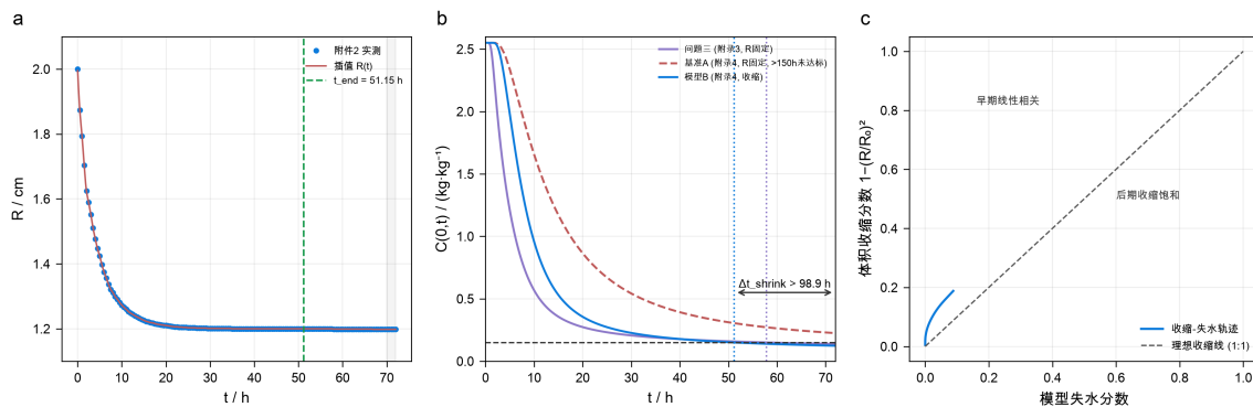
图 11 (a) 附件 2 实测半径与插值轨迹；(b) 三种设置的中心含水率对比（问题三 / 附录 4 固定半径 / 附录 4 收缩）；(c) 收缩-失水关系。
