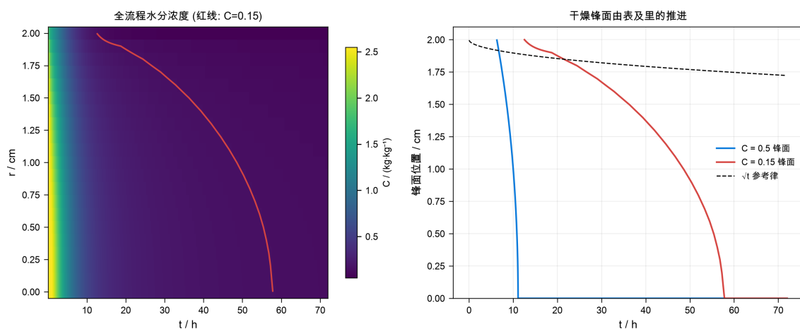
图 10 全流程水分浓度二维热图 (左) 与干燥锋面位置随时间的变化 (右，虚线为 \sqrt{t} 参考)。
