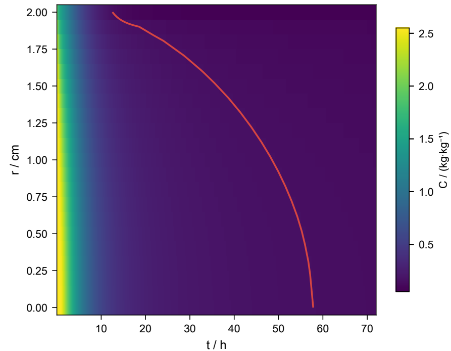
全流程水分浓度 (红线: C=0.15 )
