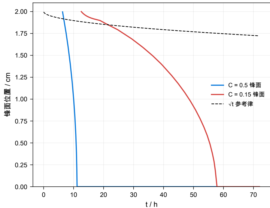
干燥锋面由表及里的推进
