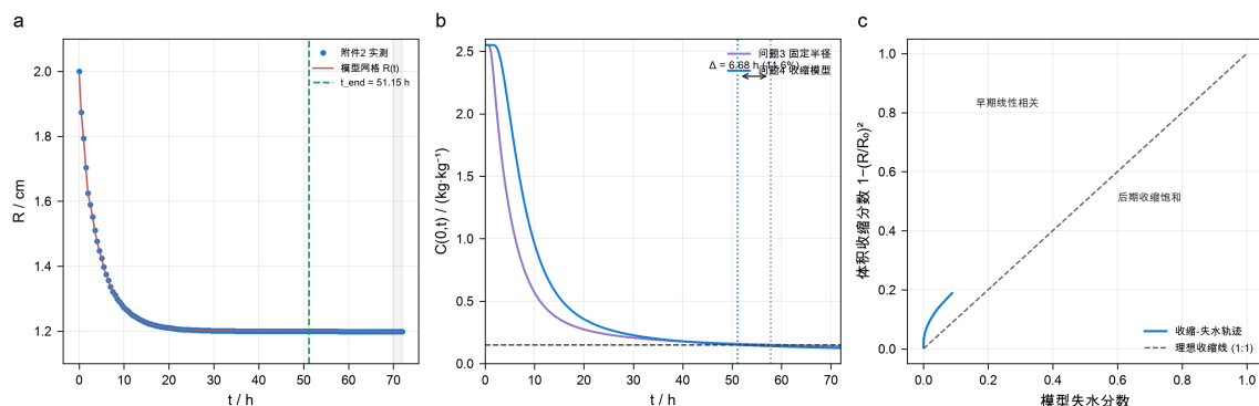
图 11 收缩干燥。(a) 附件 2 实测半径与模型使用的插值轨迹；(b) 问题三与问题四中中心含水率对比， \Delta t_{end} = 6.68 \text{ h} (11.6%)；(c) 收缩-失水关系：早期线性、后期饱和。
