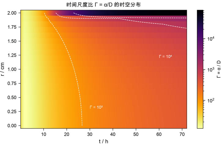
图 7 时间尺度比 \Gamma = \alpha/D 的时空分布（对数色标，虚线为等值线）。湿态 \Gamma \sim 10 、干态 \Gamma \sim 10^5 ：热湿耦合强度随干燥进程衰减。
