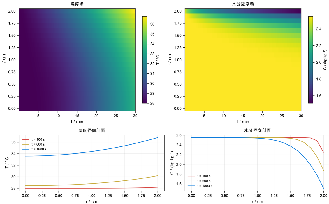
图 5 预热阶段时空演化 (二维热图, 上) 与典型时刻径向剖面 (下)。左列温度, 右列水分浓度。
