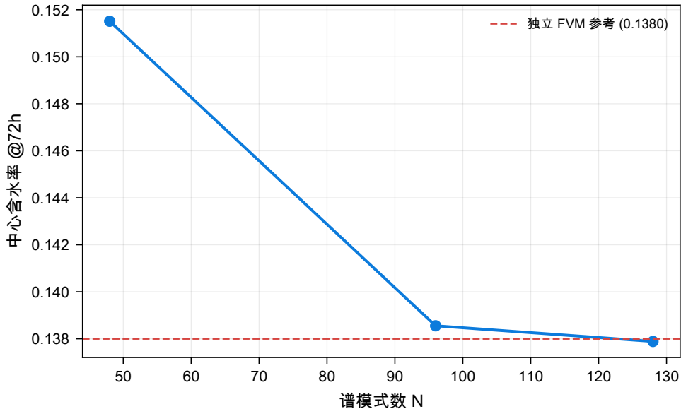
谱收敛 (问题2 干燥锋面, N=96 起收敛)
