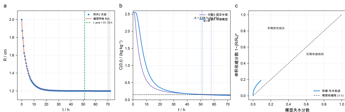
图 12 收缩干燥。(a) 附件 2 实测半径与模型使用的插值轨迹；(b) 问题三与问题四中中心含水率对比， \Delta t_{end} = 6.68 \text{ h} (11.6%)；(c) 收缩-失水关系：早期线性、后期饱和。
