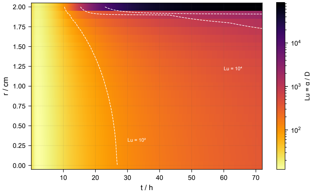
局部 Luikov 数演化 (耦合强度: 湿态强耦合 \rightarrow 干态退耦)
