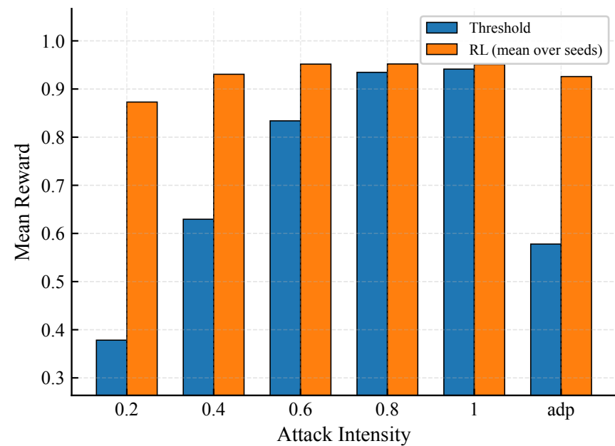
DOS - Reward
