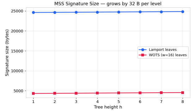
(d) MSS signature size vs. height.
