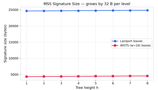
(d) MSS signature size vs. height.
