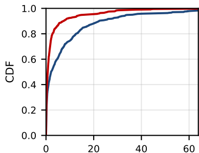
(d) RMSE
