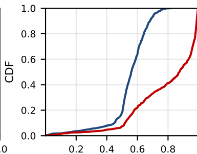
(b) NNSE
