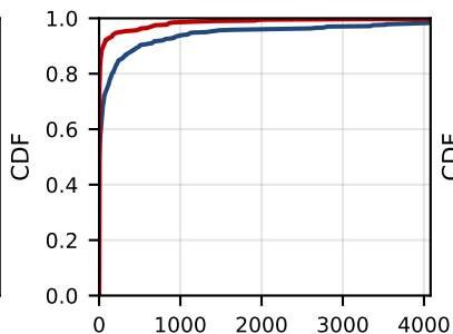
(e) MSE
