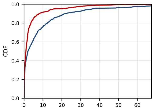
(d) RMSE
