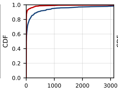
(e) MSE
