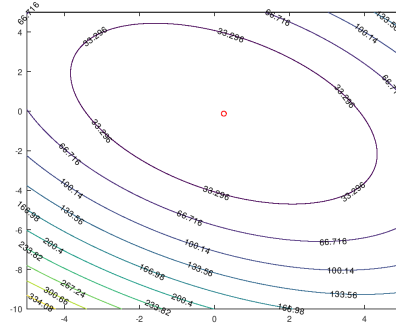
FIGURA 5. Curvas de nivel de J(x_1, x_2) = 5/2x_1^2 + 2x_2^2 + 2x_1x_2 - x_1 .
