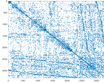
FIGURA 2. Estructura de la matriz A : se observa que es rala y simétrica.
