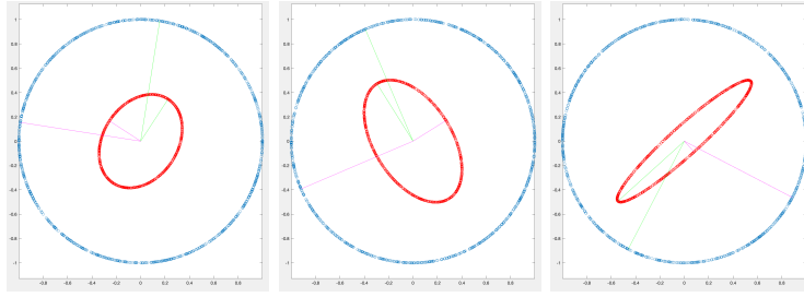
FIGURA 2. Elípses obtenidas por el mapeo del círculo unitario a través de matrices generales.
