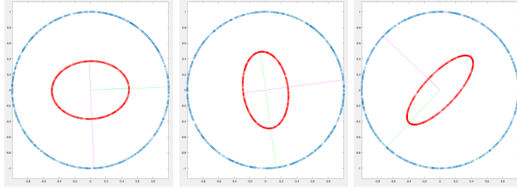
FIGURA 1. Elípses obtenidas por el mapeo del círculo unitario a través de matrices simétricas.
