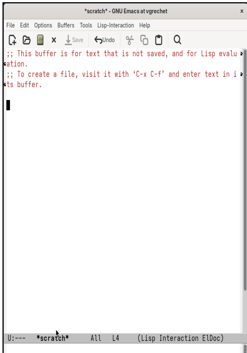
Рисунок 2.10: Переключение буфера
