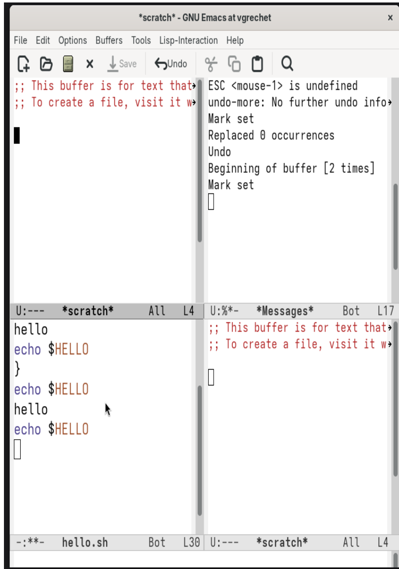
Рисунок 2.11: Четыре буфера
