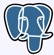
Postgres
