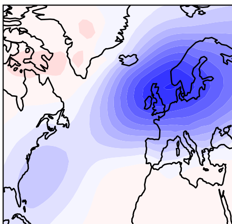
MPI-ESM1-2-LR
