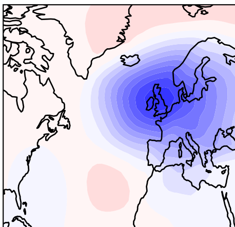
GISS-E2-1-G
