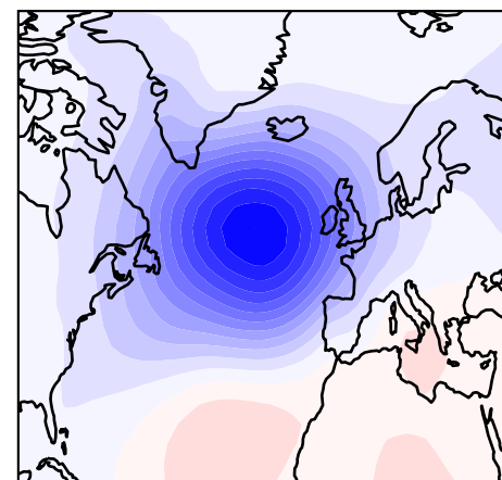
MIROC6
