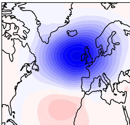
MPI-ESM1-2-LR
