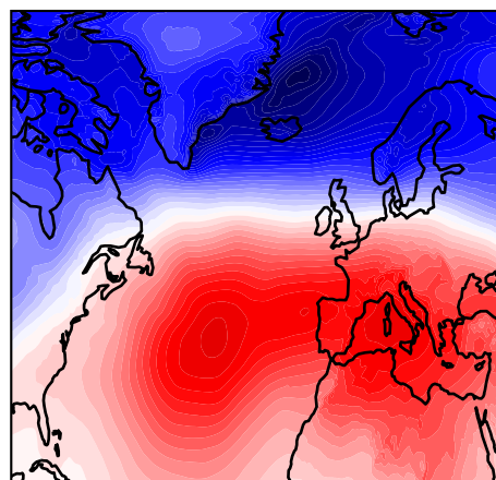
era5
