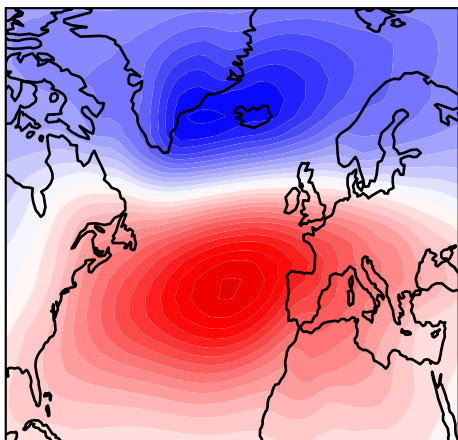
NorESM2-LM
