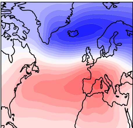
GISS-E2-1-G
