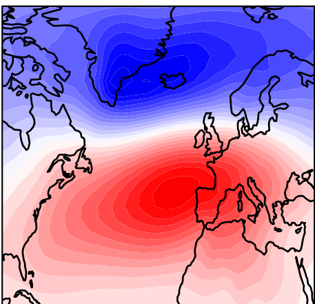
MPI-ESM1-2-LR
