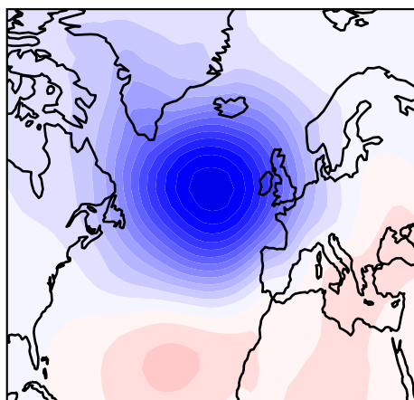
NorESM2-LM
