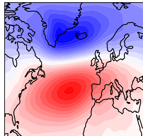
MIROC6
