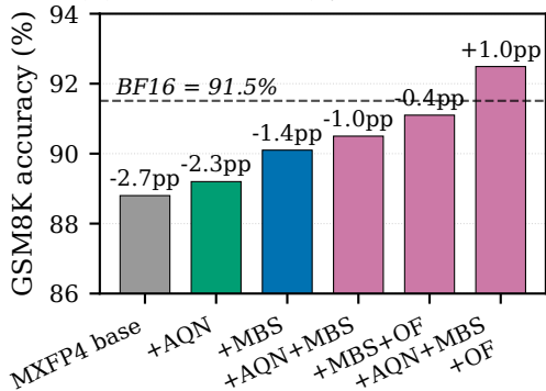
(a) MoE W4A4 (Qwen3-30B-A3B)
