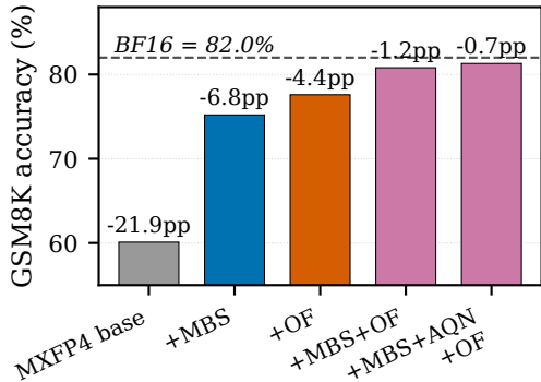
(b) Dense W4A4 (Qwen2.5-3B)
