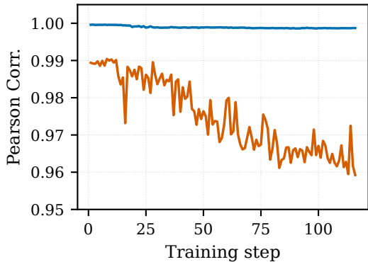
(a) GSM8K (~280-token)
