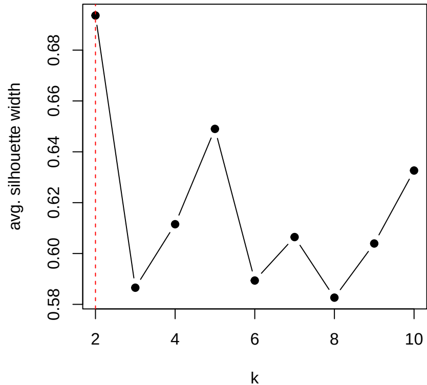
VIC -- cs (euclidean)
