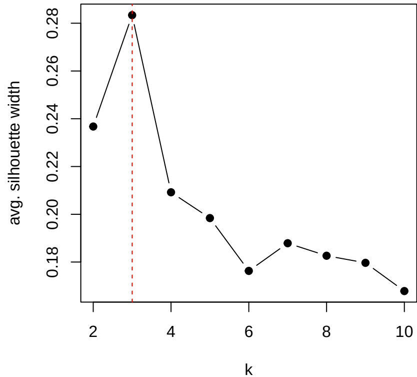
VIC -- gc (manhattan)
