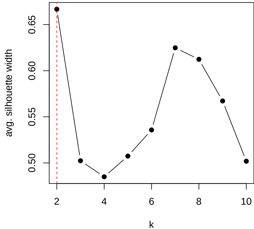
VIC -- mk (manhattan)
