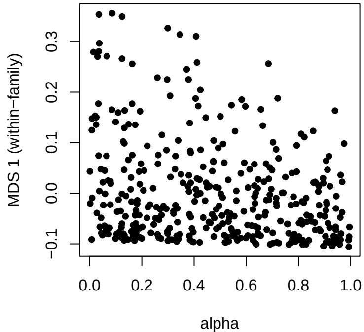
bc / glmnet
