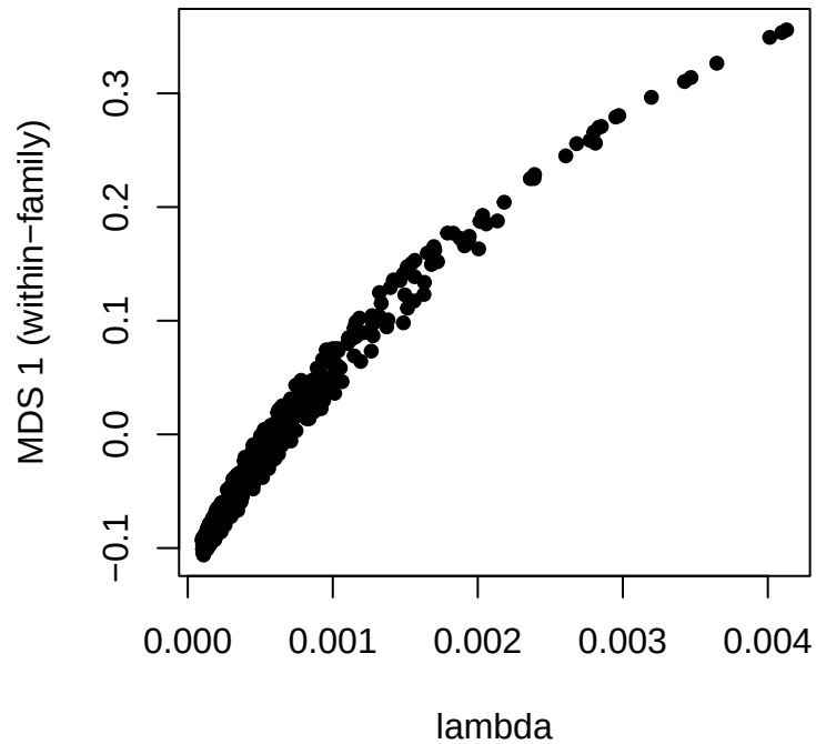
bc / glmnet
