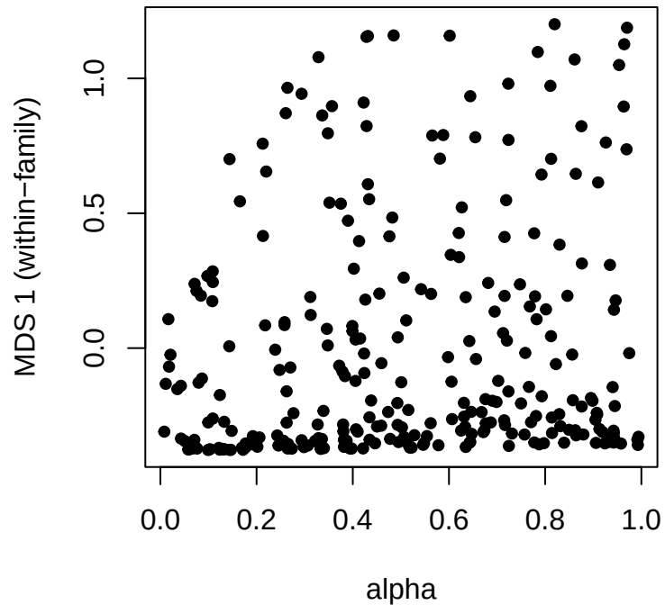
cs / glmnet
