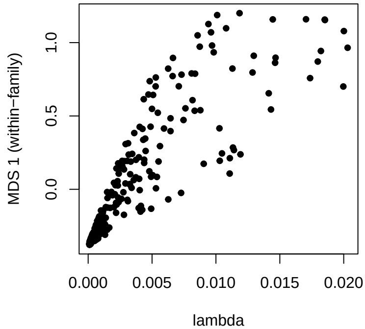
cs / glmnet
