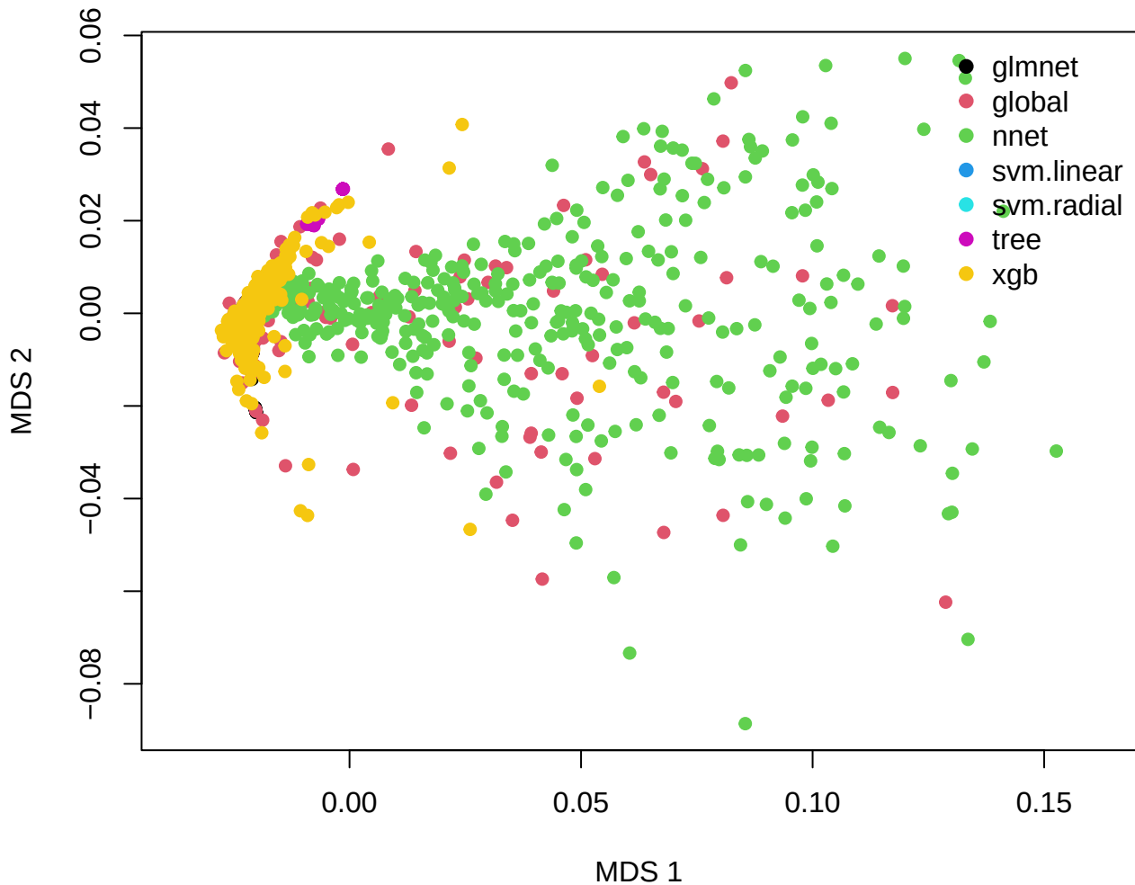
VIC MDS -- cs.bin (euclidean)
