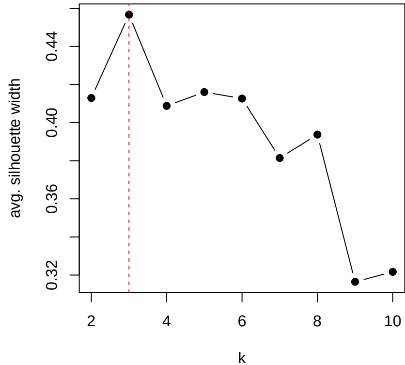
VIC -- fc.bin (manhattan)
