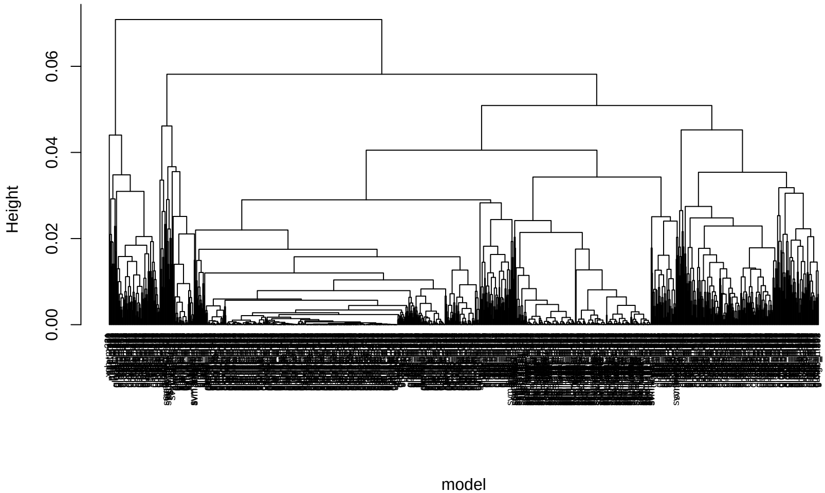
VIC dendrogram -- fc.bin (manhattan)
