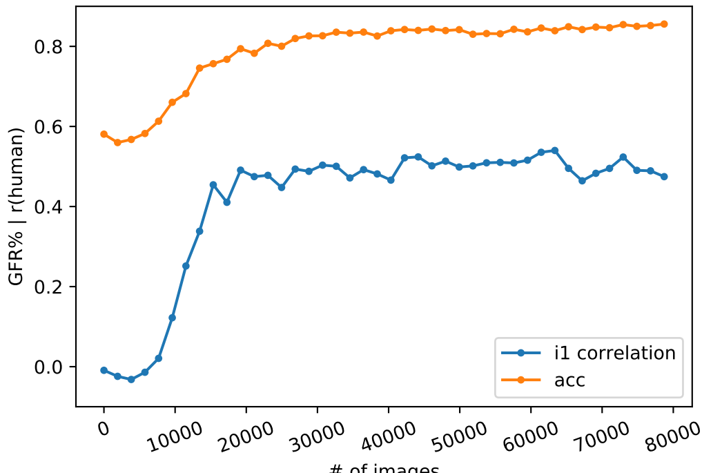
Elias-Neptune fine-tuning, 1 epoch
