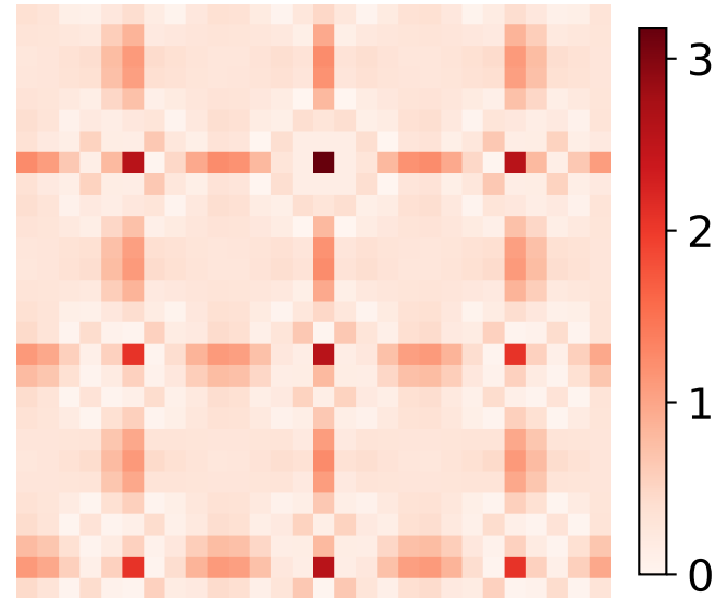
1-body Appx. Error
