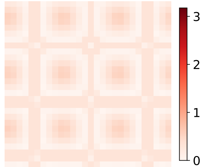
2-body Appx. Error
