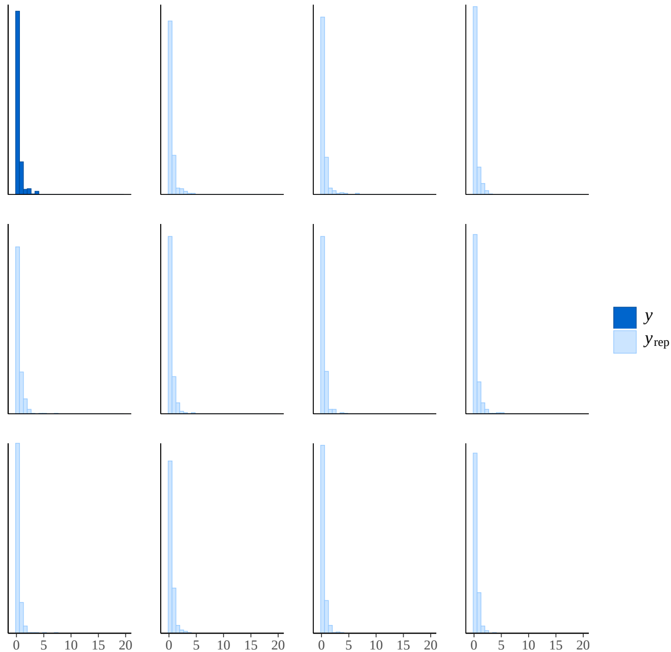
BWWA
