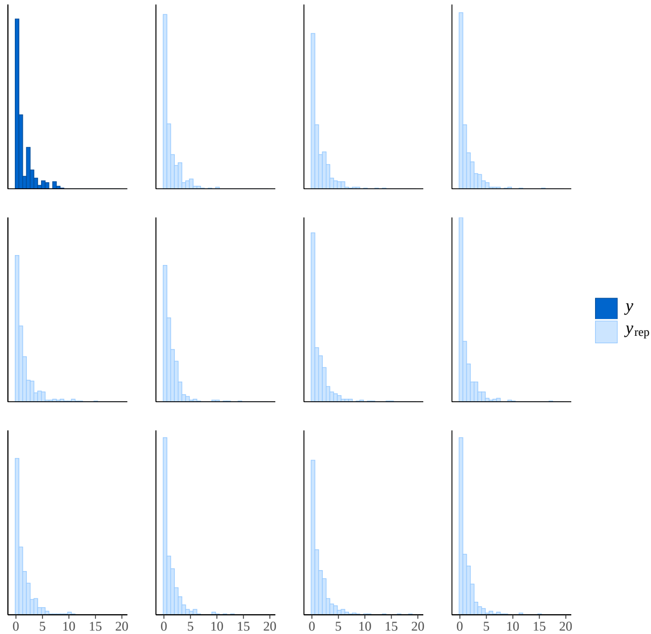
RBNU
