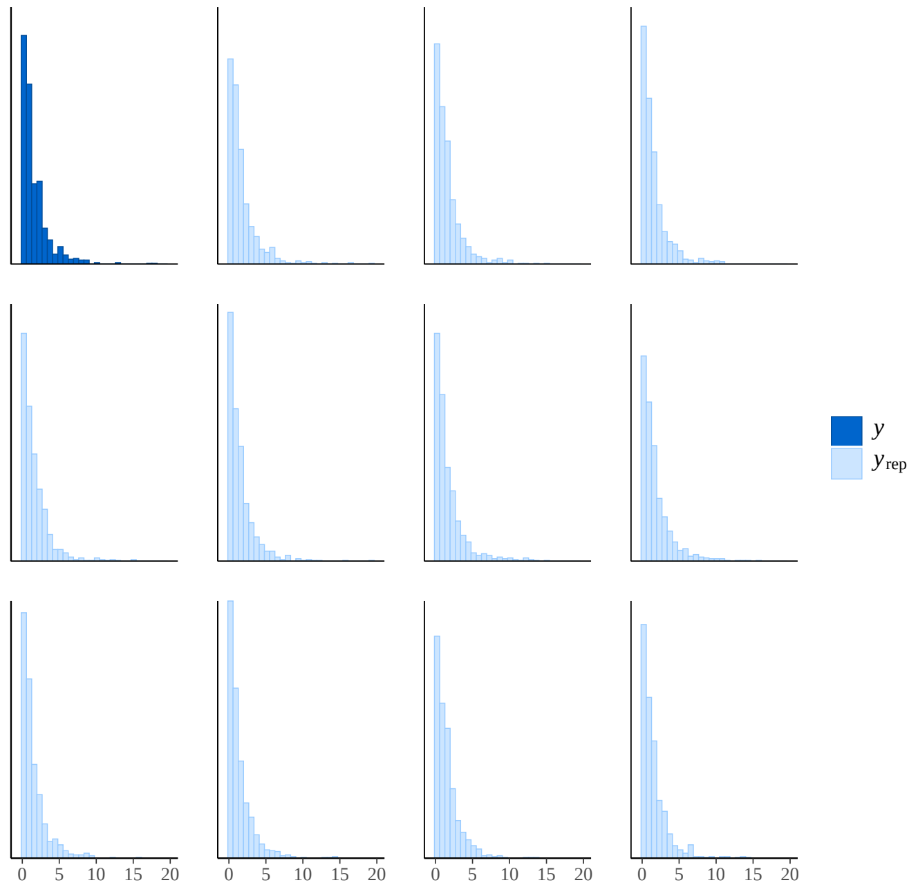
BEWR
