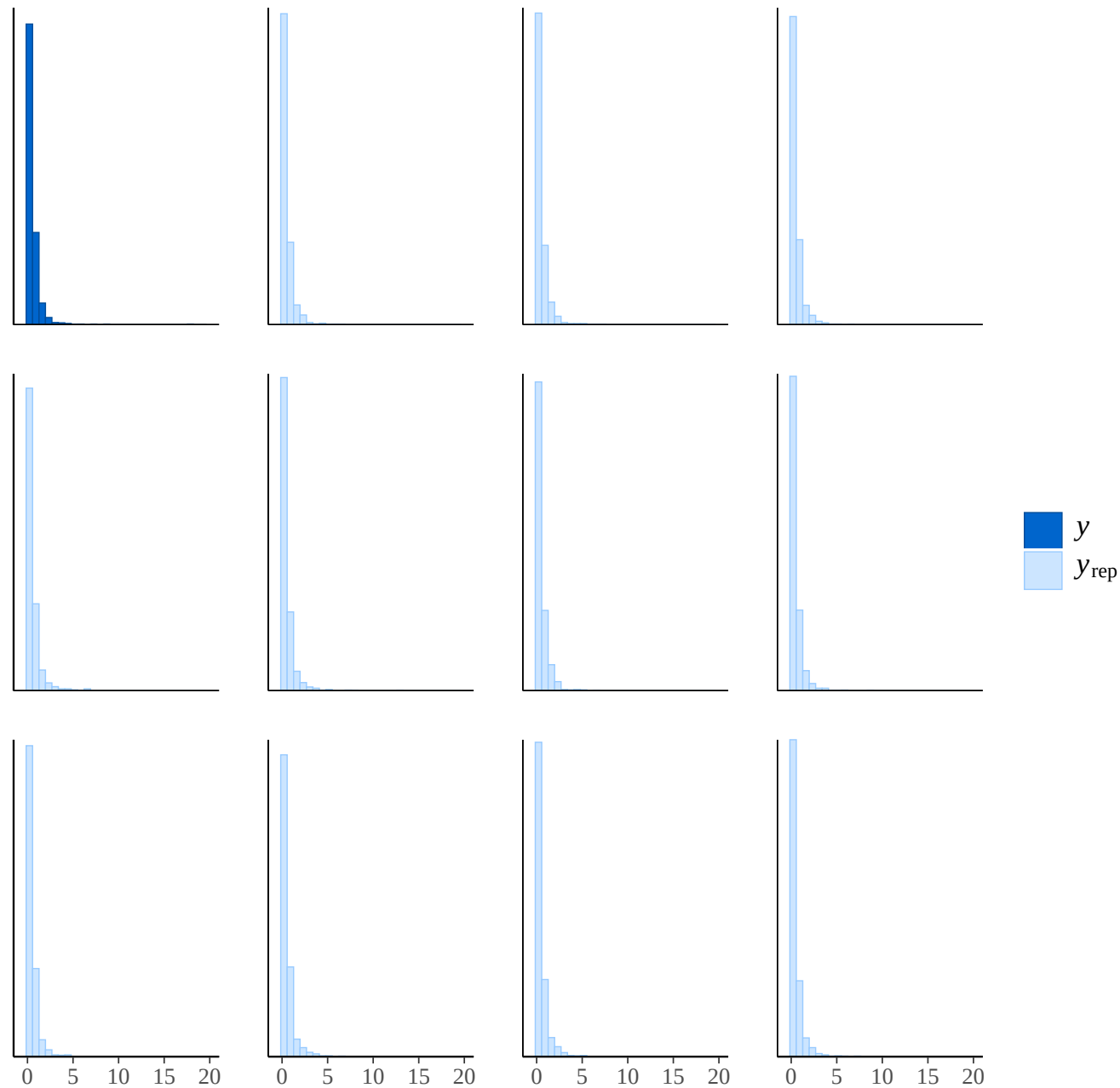
GRCA
