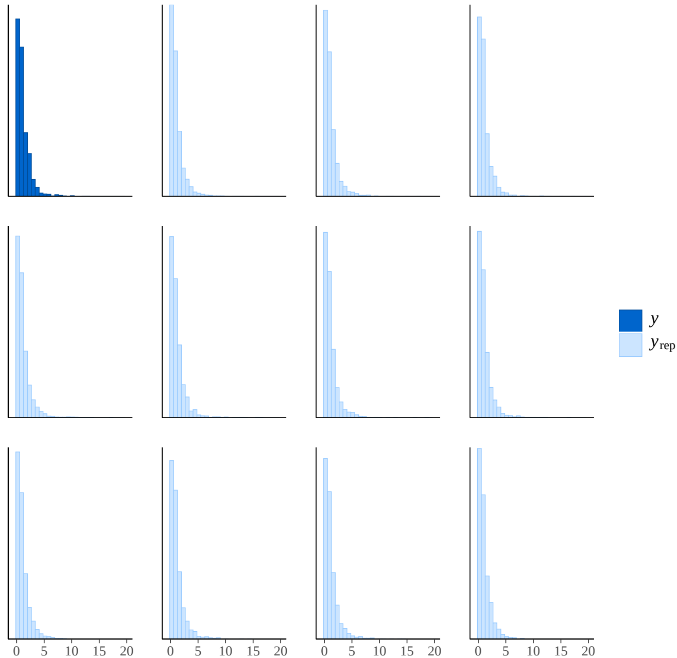
SOSP
