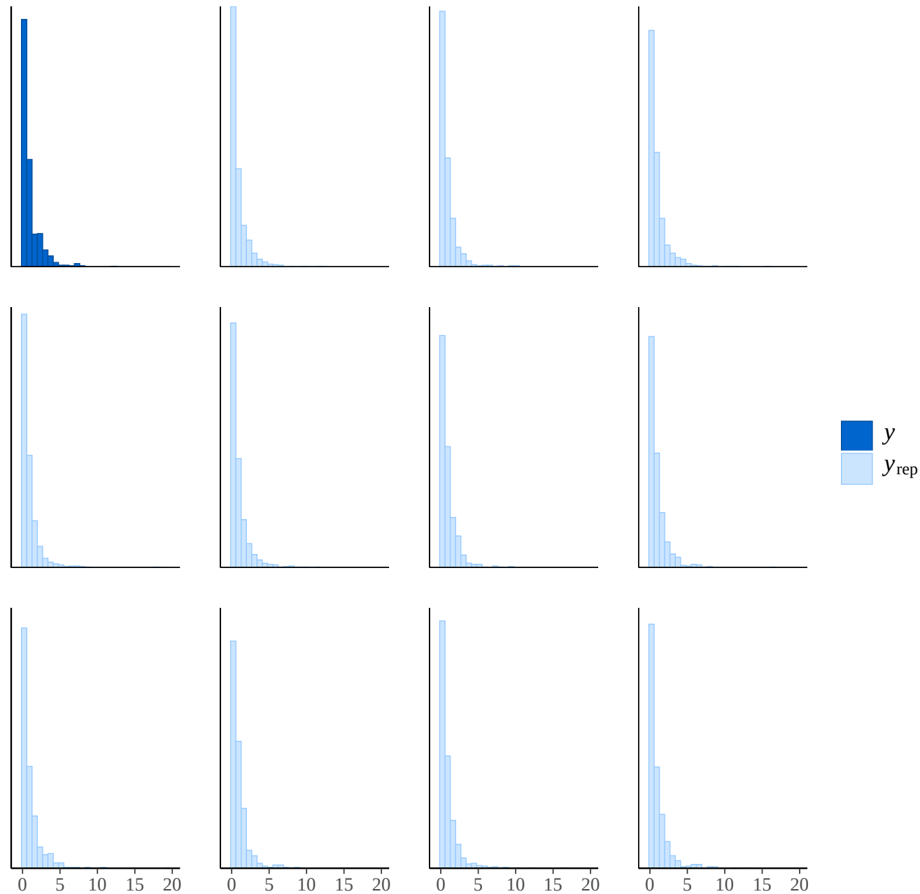
SPTO
