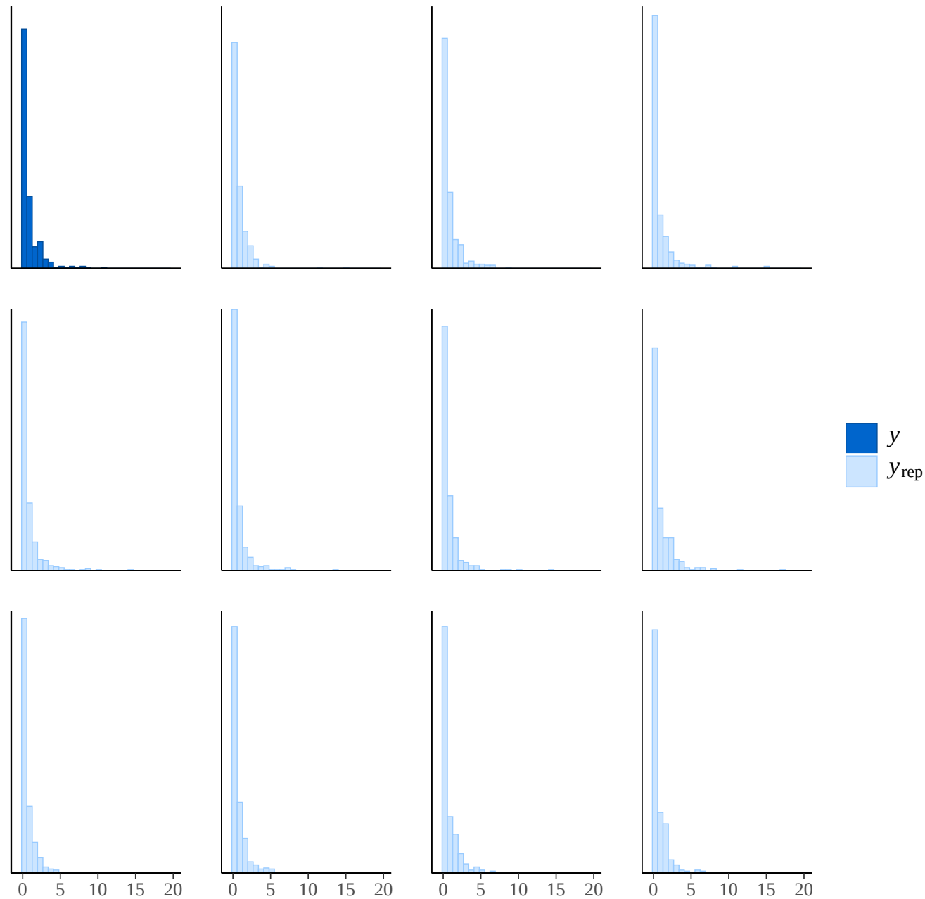
HOFI
