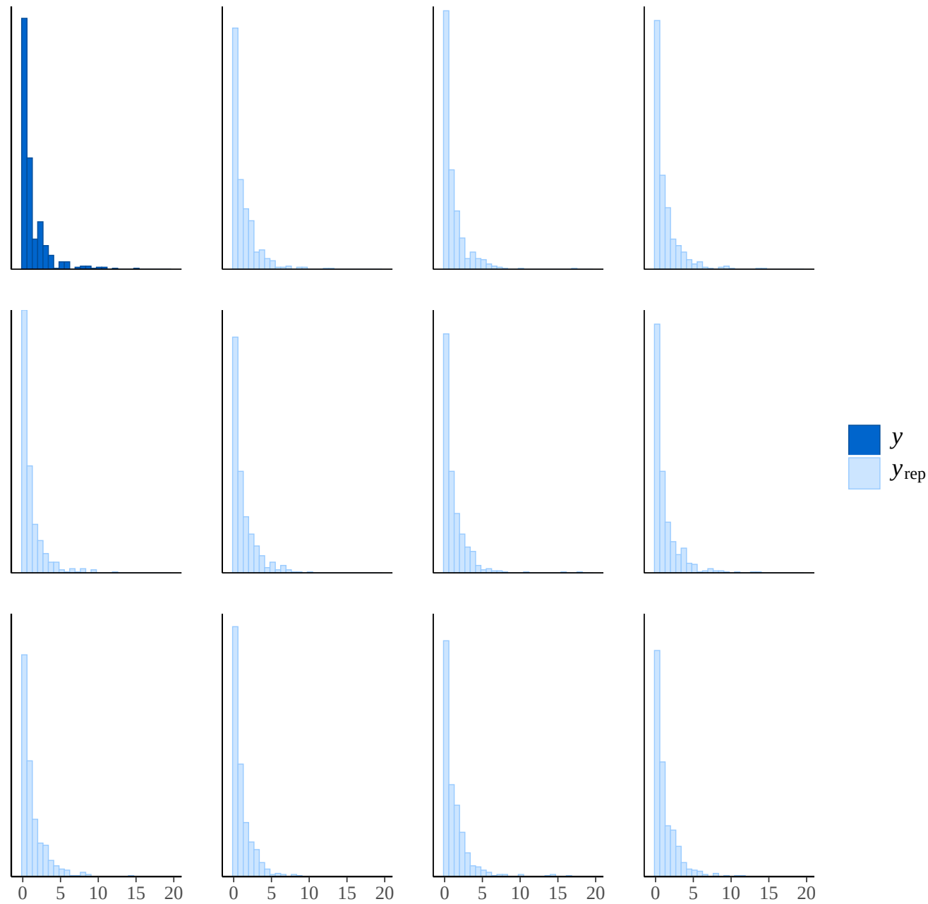
BRCR
