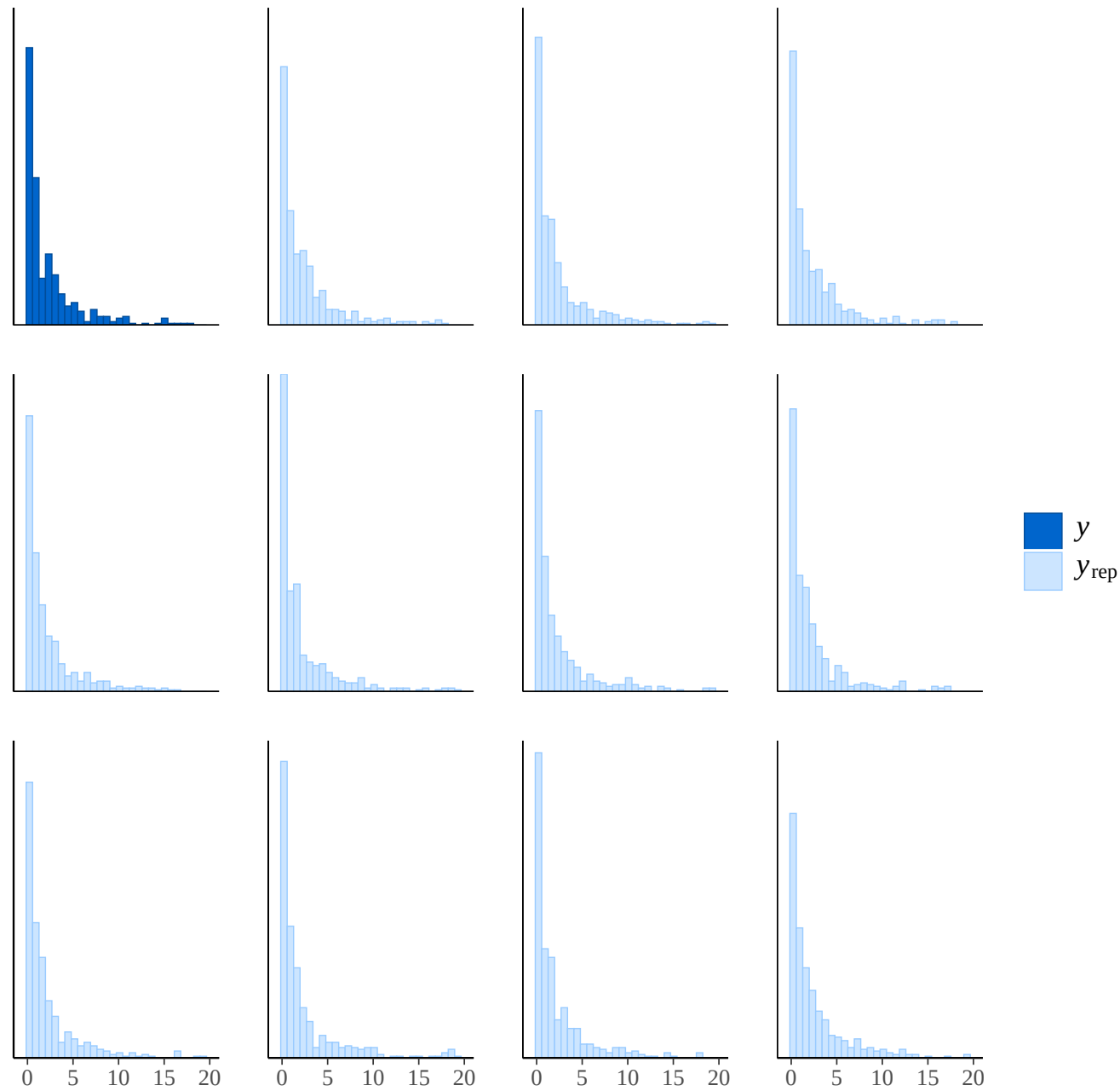
GCKI
