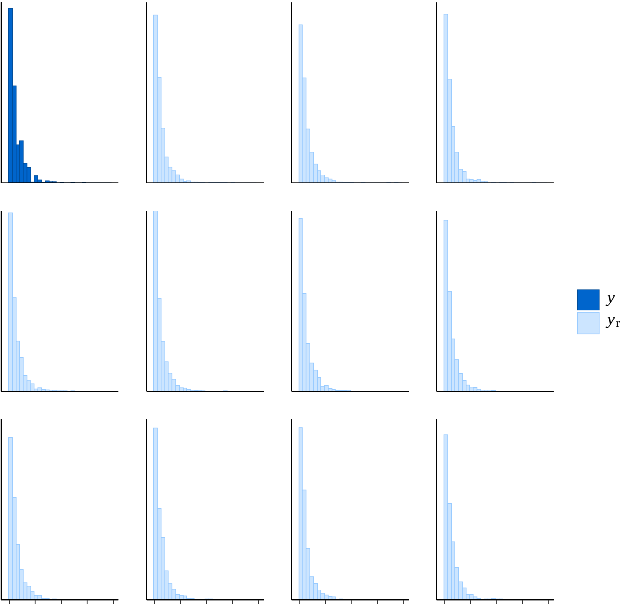
CARW
