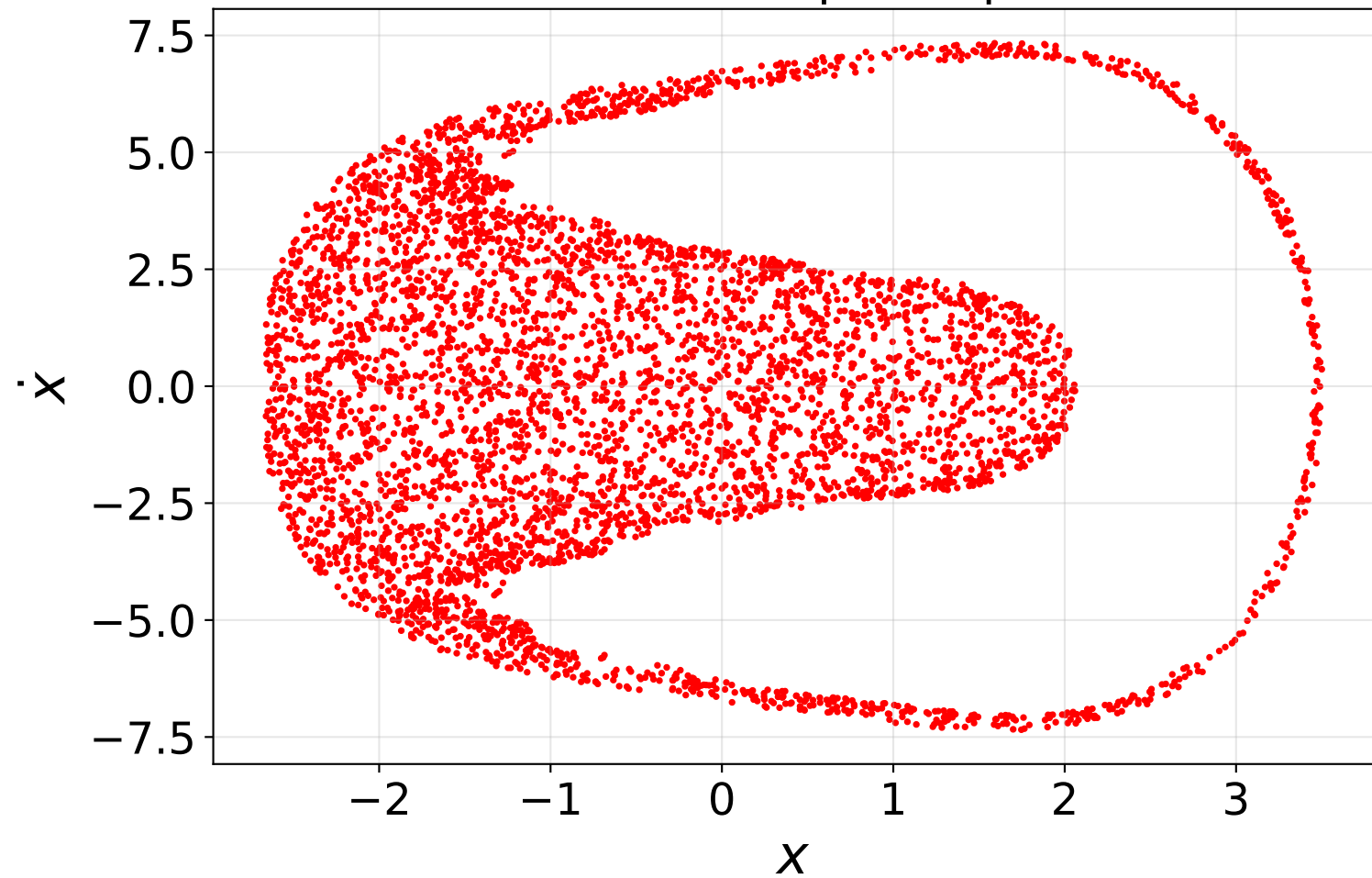
Stroboscopic map
