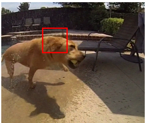
PhaseNet-big
