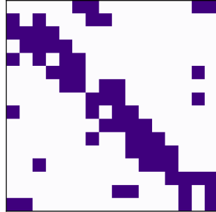
Kucuk-dunya (kapsama 0.61)
