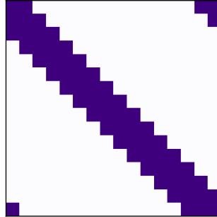
Halka (kapsama 0.44)
