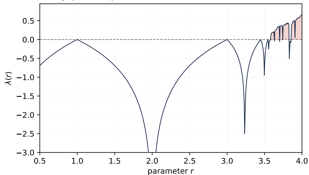
(d) Lyapunov exponent ( \lambda > 0 : chaotic)
