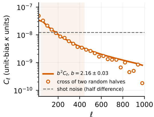
LRG 0.8-1.1
