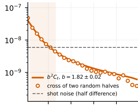
QSO 1.1-1.6
