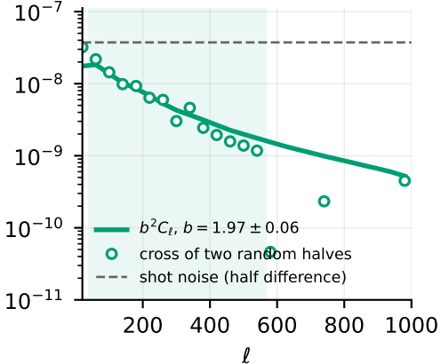
QSO 1.1-1.6
