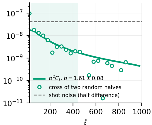
QSO 0.8-1.1
