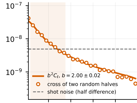
QSO 1.6-1.75
