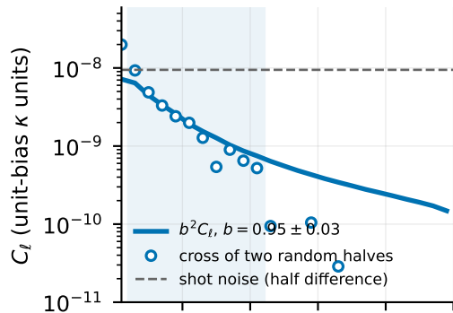
LRG 0.8-1.1
