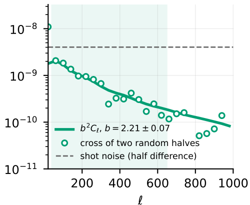
QSO 1.6-1.75
