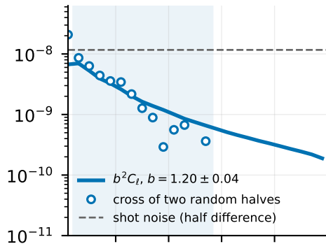
QSO 0.8-1.1
