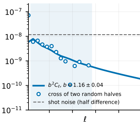
QSO 0.8-1.1
