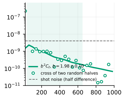
QSO 1.6-1.75
