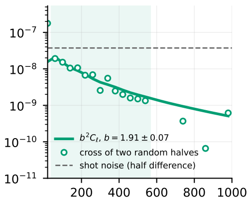
QSO 1.1-1.6
