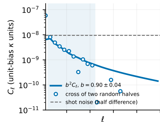
LRG 0.8-1.1
