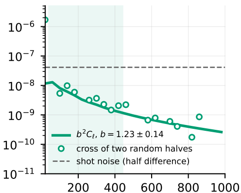
QSO 0.8-1.1
