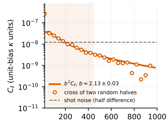
LRG 0.8-1.1
