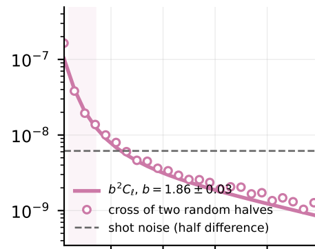
BOSS 0.1-0.4
