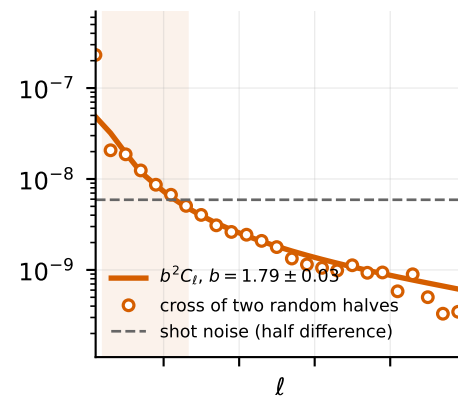
QSO 1.1-1.6
