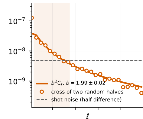
QSO 1.6-1.75
