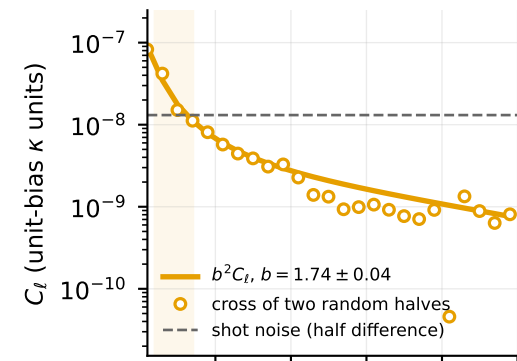
BGS 0.1-0.4
