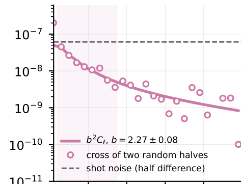
BOSS 0.6-0.8
