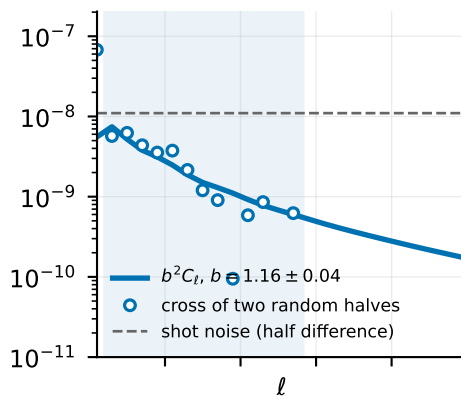
QSO 0.8-1.1
