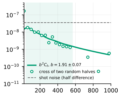
QSO 1.1-1.6
