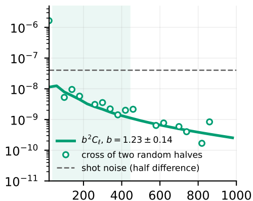
QSO 0.8-1.1
