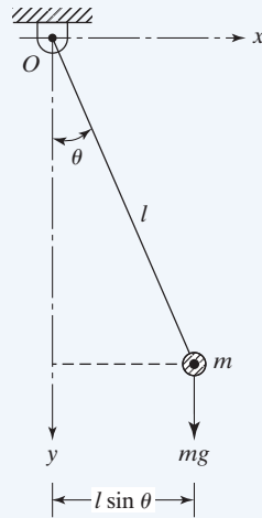
Simple pendulum.
