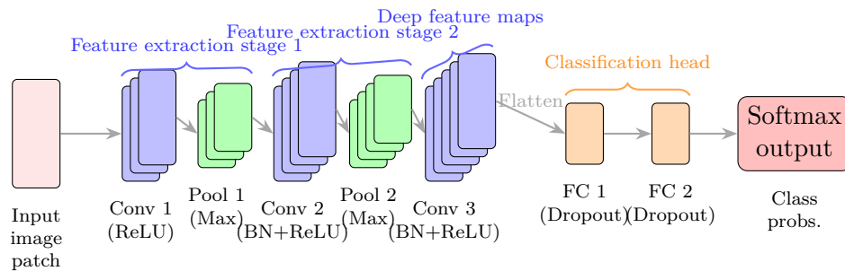
Figura 4.1: Architettura schematica di una rete neurale convoluzionale (CNN) applicata alla classificazione di immagini istopatologiche. Un patch dell'immagine di input viene elaborato attraverso successivi strati convoluzionali e di pooling che estraggono caratteristiche gerarchiche di crescente astrazione. Il vettore di caratteristiche risultante viene passato a strati completamente connessi e a uno strato di output softmax che produce le probabilità di classe. Conv: strato convoluzionale; Pool: strato di pooling; FC: strato completamente connesso.
