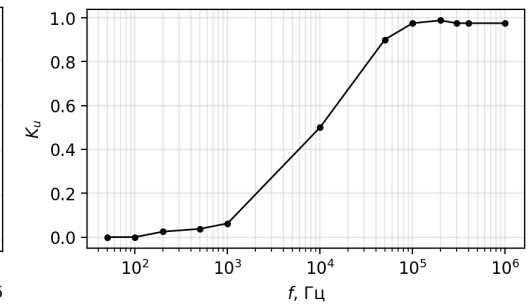
K_u(f) в логарифмическом масштабе
