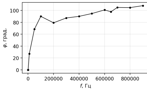
\varphi(f) в линейном масштабе
