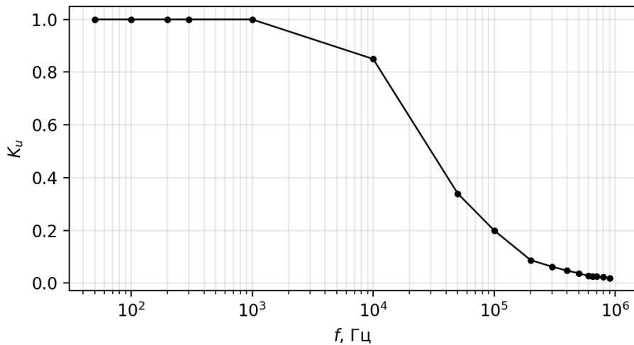
K_u(f) в логарифмическом масштабе осей
