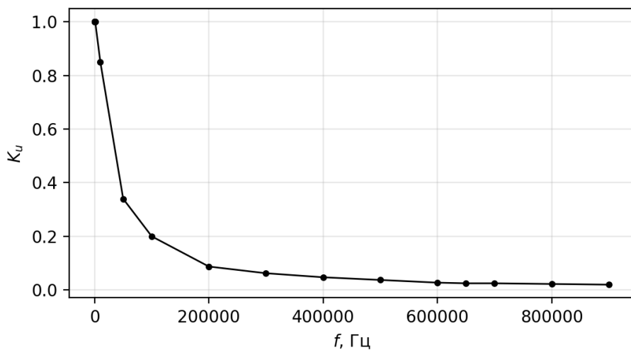
K_u(f) в линейном масштабе осей
