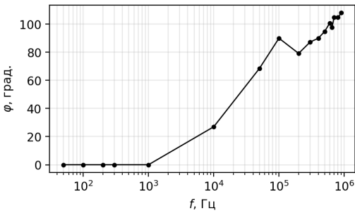
\varphi(f) в логарифмическом масштабе
