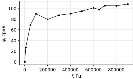
\varphi(f) в линейном масштабе
