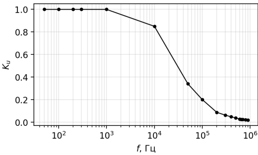
K_u(f) в логарифмическом масштабе
