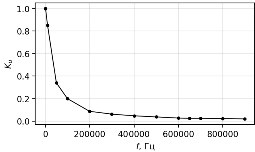
K_u(f) в линейном масштабе
