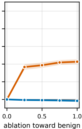
CICIoT2023
