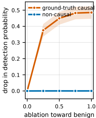
5G-NIDD
