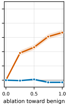
CICIoMT2024
