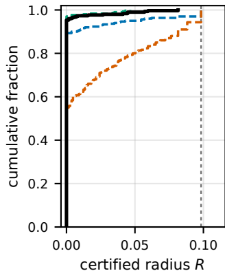
5G-NIDD
