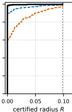
CICIoT2023
